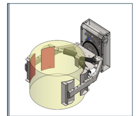
Pince électrique avec bloc de rotation 360°
